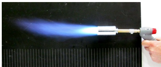
Admission d'air ouvert en grand
